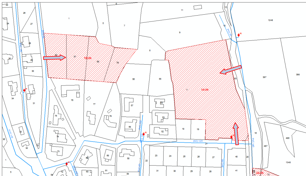
↖ Carte 4 : Raccordement AEP – secteur AU (Nord du centre-bourg)
