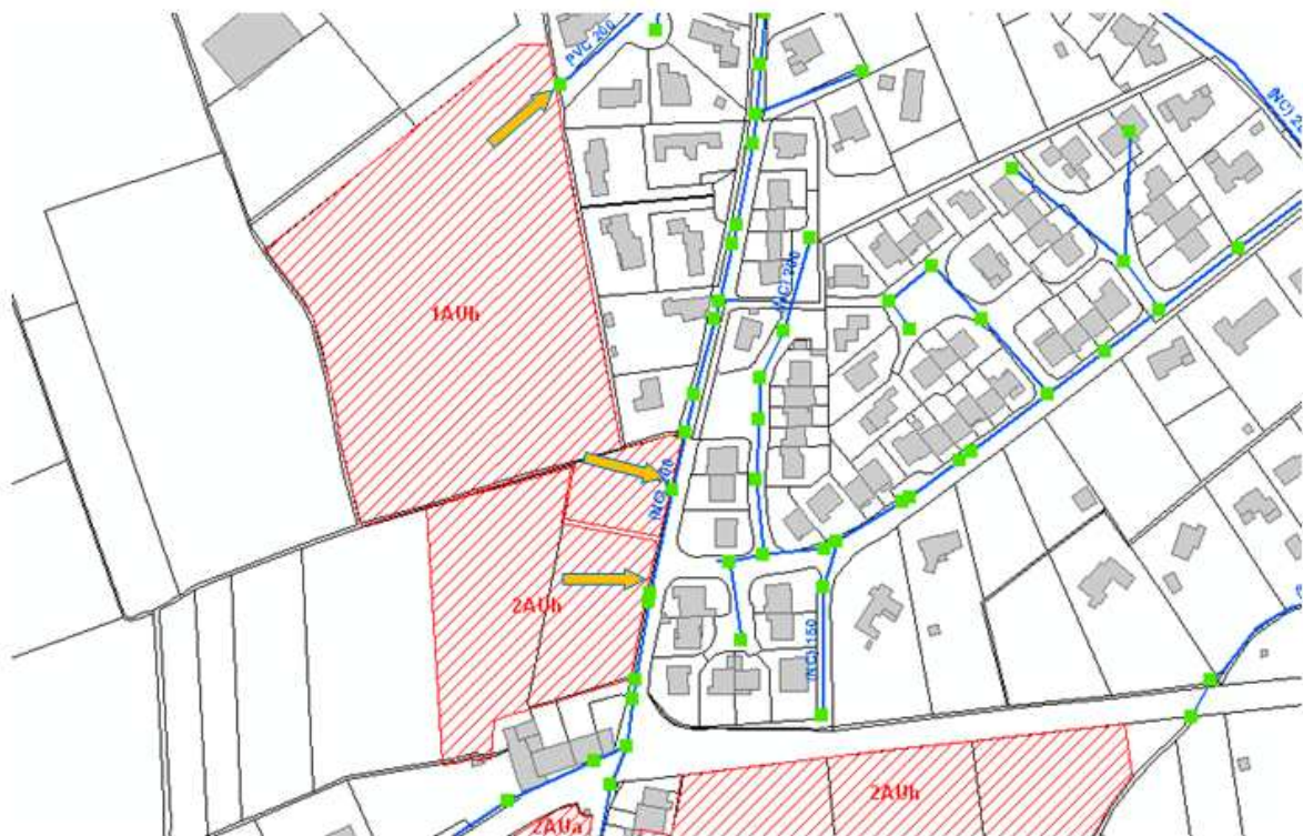
↪ Carte 7 : Raccordement EU – secteur AU (coté nord de l'avenue de la Mer)
