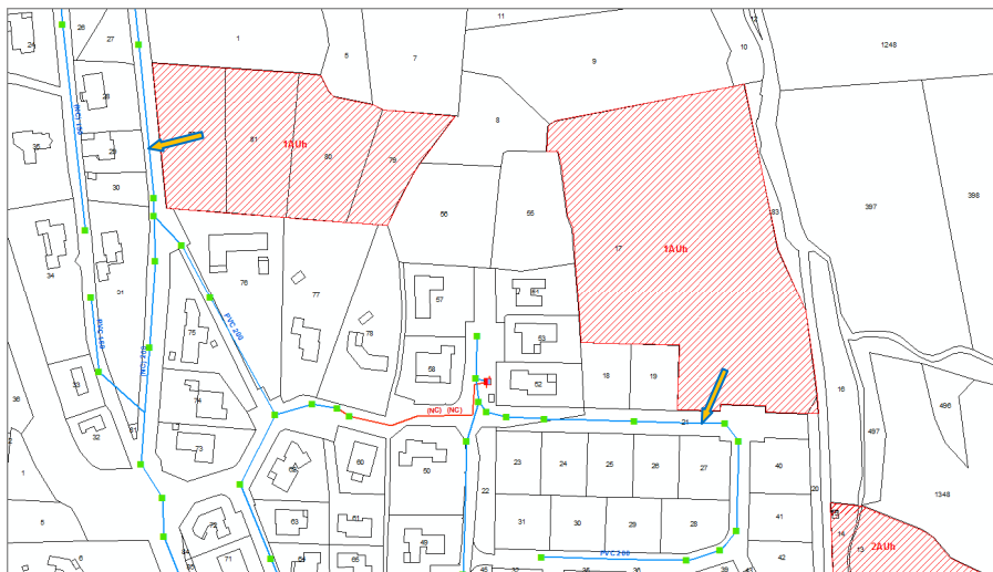
↳ Carte 10 : Raccordement EU – secteur AU (Nord du centre-bourg)
