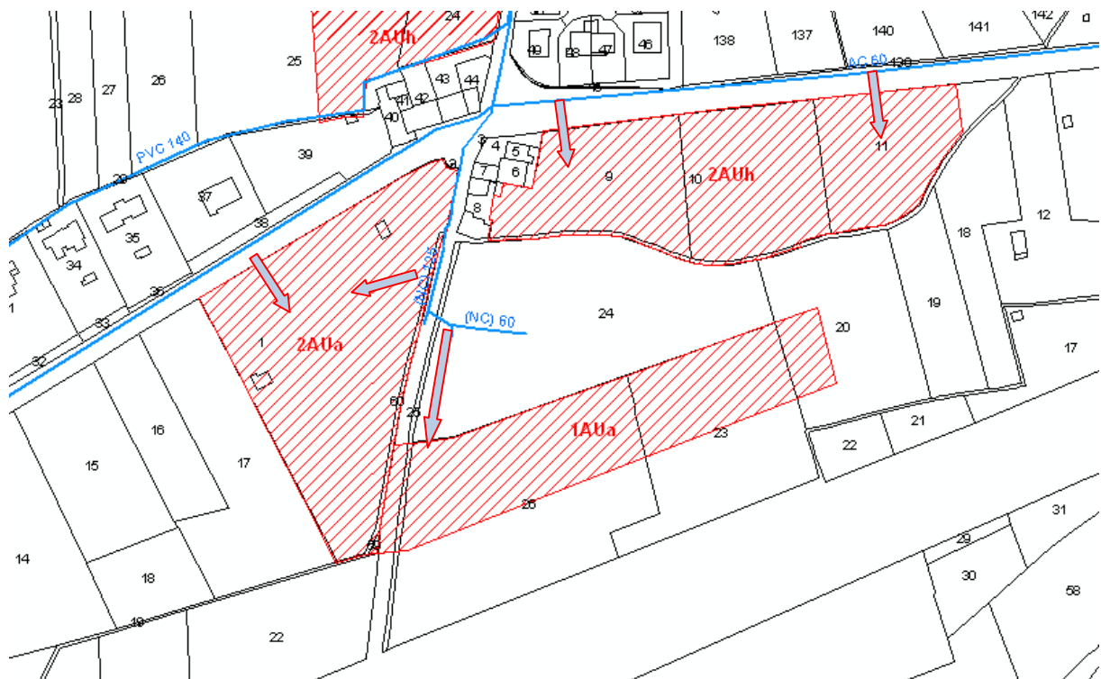
↶ Carte 2 : Raccordement AEP – secteur AU (coté sud de l'avenue de la Mer)
